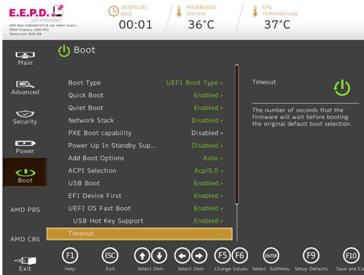
Fig. 76: Boot Menu 1
